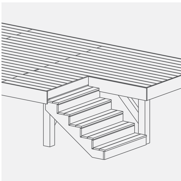
EN OPTION, ESCALIER TYPE DIEPPE
