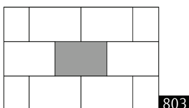
1 module de pose : 0,240 m 2 60 x 40 1 pièce 100 % de la surface
