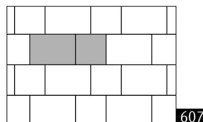
1 module de pose : 0,064 m 2 16 x 16 1 pièce 40% de la surface 24 x 16 1 pièce 60% de la surface
